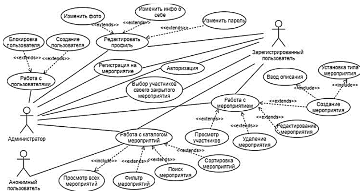
Рисунок 3 – Пример диаграммы вариантов использования web-системы в нотации UML для event-менеджмента
