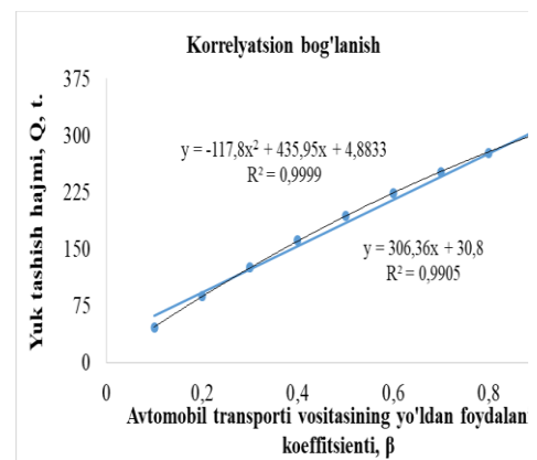
e. Yuk tashish hajmining yo'ldan foydalanish koeffitsientiga bog'liqligi grafigi
