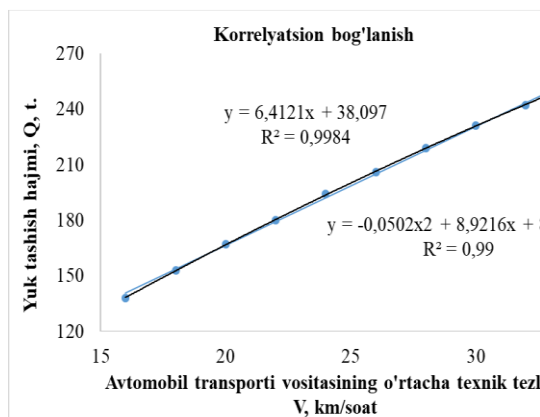
d. Yuk tashish hajmining o'rtacha texnik tezligiga bog'liqligi grafigi
